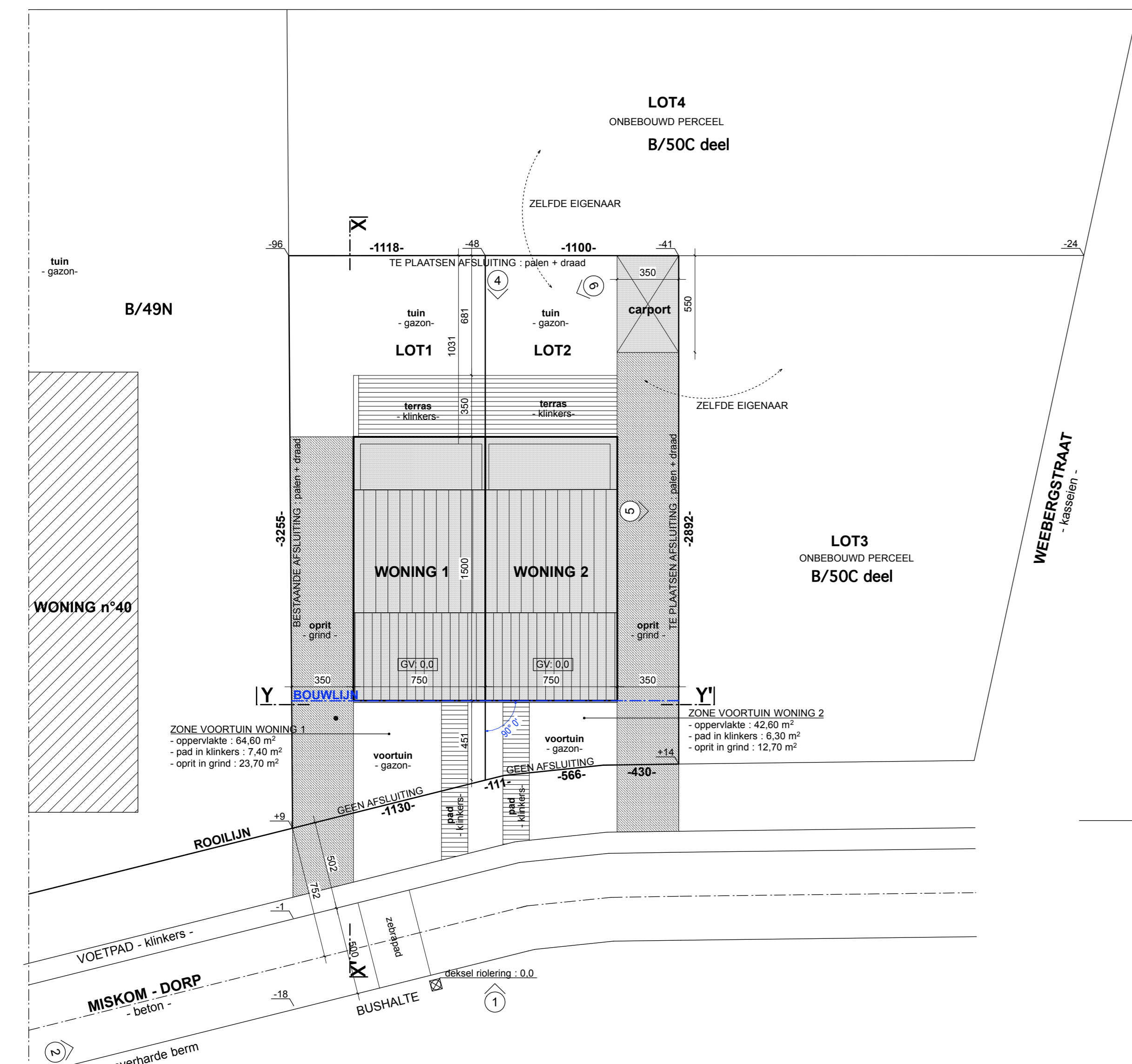
INPLANTINGSPLAN schaal : 1/200
